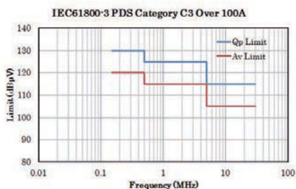
図14 100 Aを超える装置の伝導エミッション許容値
