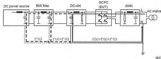
図3 一般的なパワーコンディショナーセットアップ図
