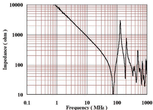
図9 長さ30 cmの電源線コモンモードインピーダンス
