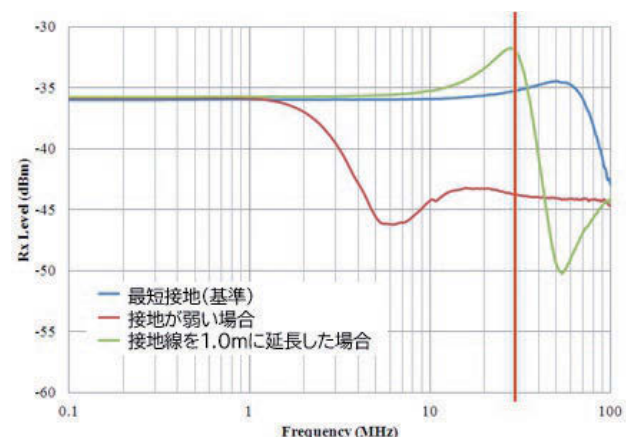
図13 ハイインピーダンスプローブの接地方法による測定結果の変化
