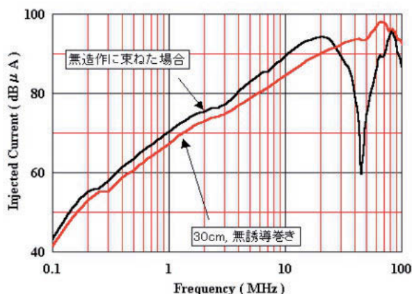
図10 ケーブル処理方法の差による妨害波注入レベルの変化
