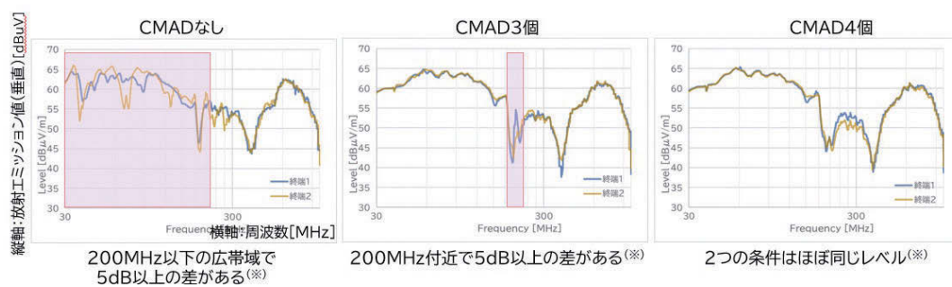
図7 CMADの本数を増加させた時の放射エミッションの変化
