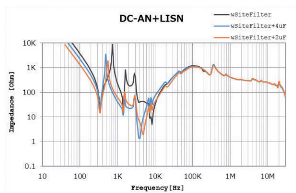
図6 全DC電力供給チェーン内の実効全CMインピーダンス結果
