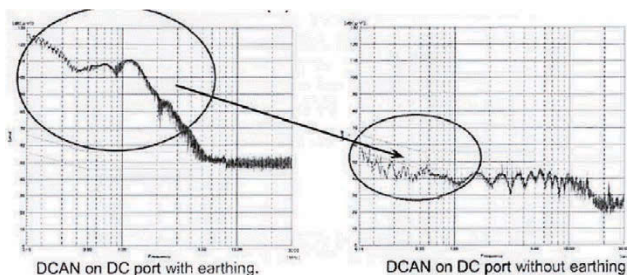
図4 過剰な伝導ノイズが発生した事例
