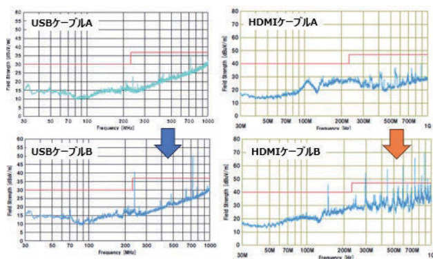
図11 ケーブルの違いによるエミッションレベルの変化(USBとHDMI)
