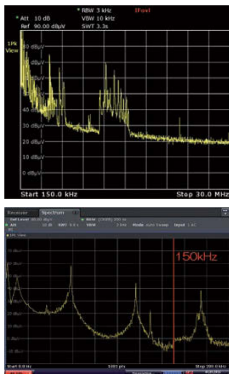
図15 規程周波数外に過大な伝導ノイズが発生した例
