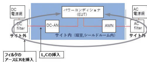
図5 検証を実施したセットアップ図
