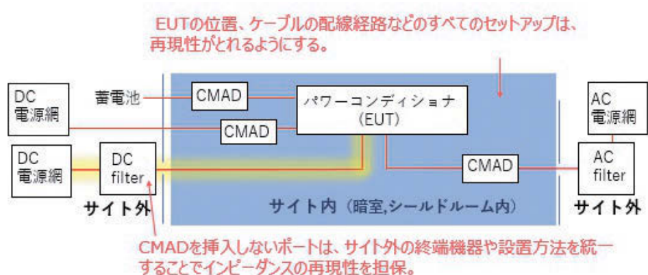
図8 CMADを使用する際の注意点
